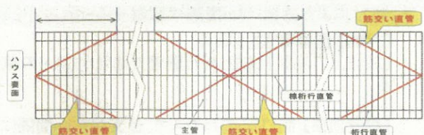
筋交いによる妻面の補強方法事例
