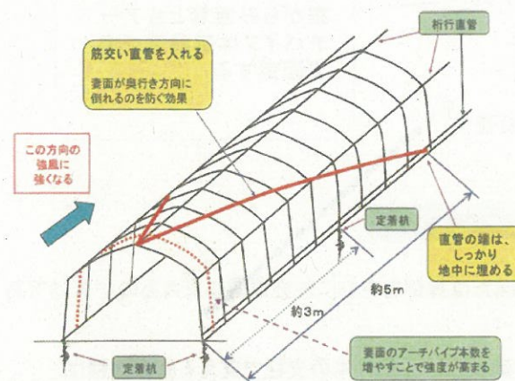
筋交いによる妻面の補強方法事例
