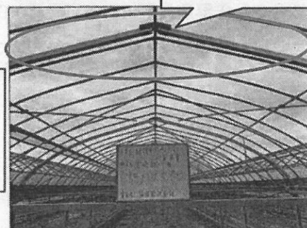
補強合掌の追加
